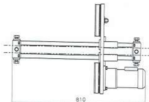
寸法図
